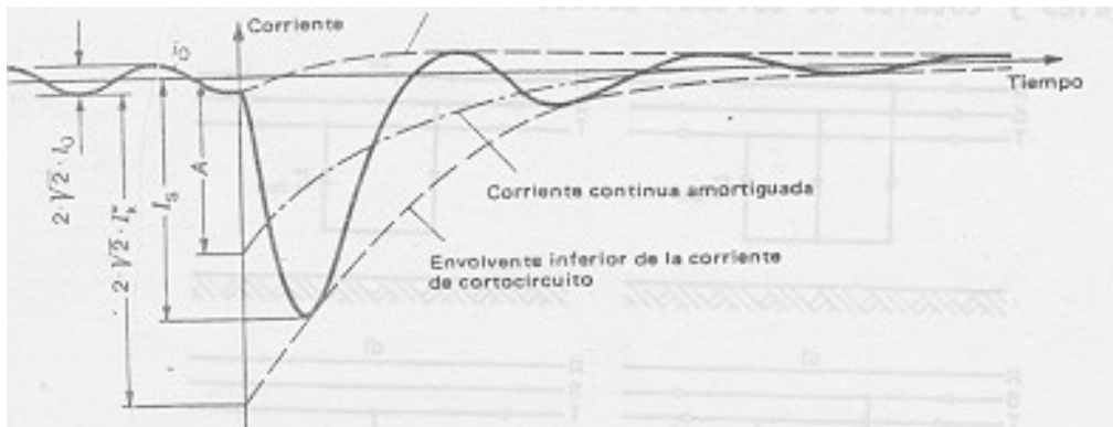
Corriente de cortocircuito de un motor asíncrono de baja tensión, para la fase con el momento de conexión más desfavorable.
